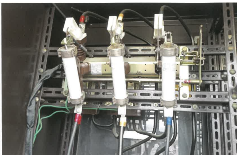
落雷による高圧パワーヒューズの溶断と放電の痕跡
